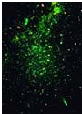
Imagen 1: Constelación estelar
