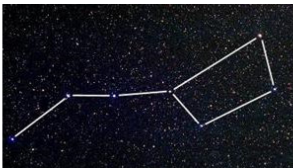
Imagen 5: Osa Mayor
