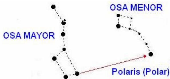
Imagen 7: Posición Constelaciones
